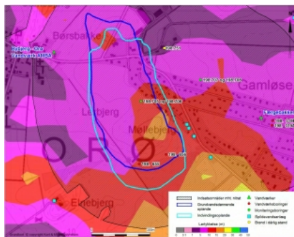
Lertykkelse og oplande - Bybjerg-Orø Vandværk.
